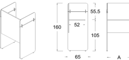
PUESTO DE CONSULTA ALTO CON FRONTAL MADERA Y LATERALES MIXTOS.
