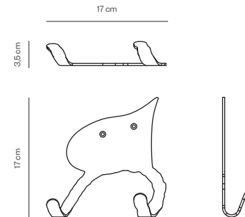
Hook N. 4
